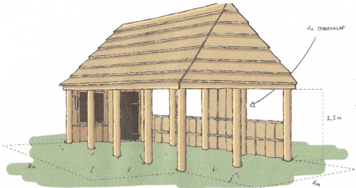
Illustration af bålhytten
