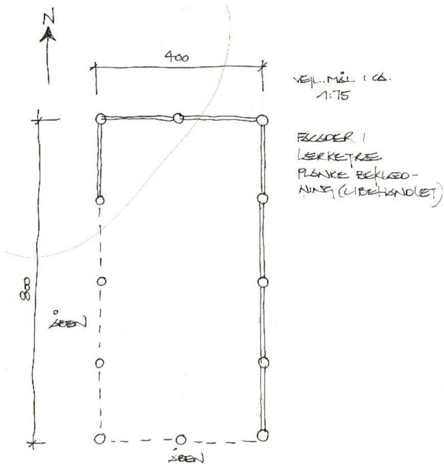
Plantegning af bålhytten
